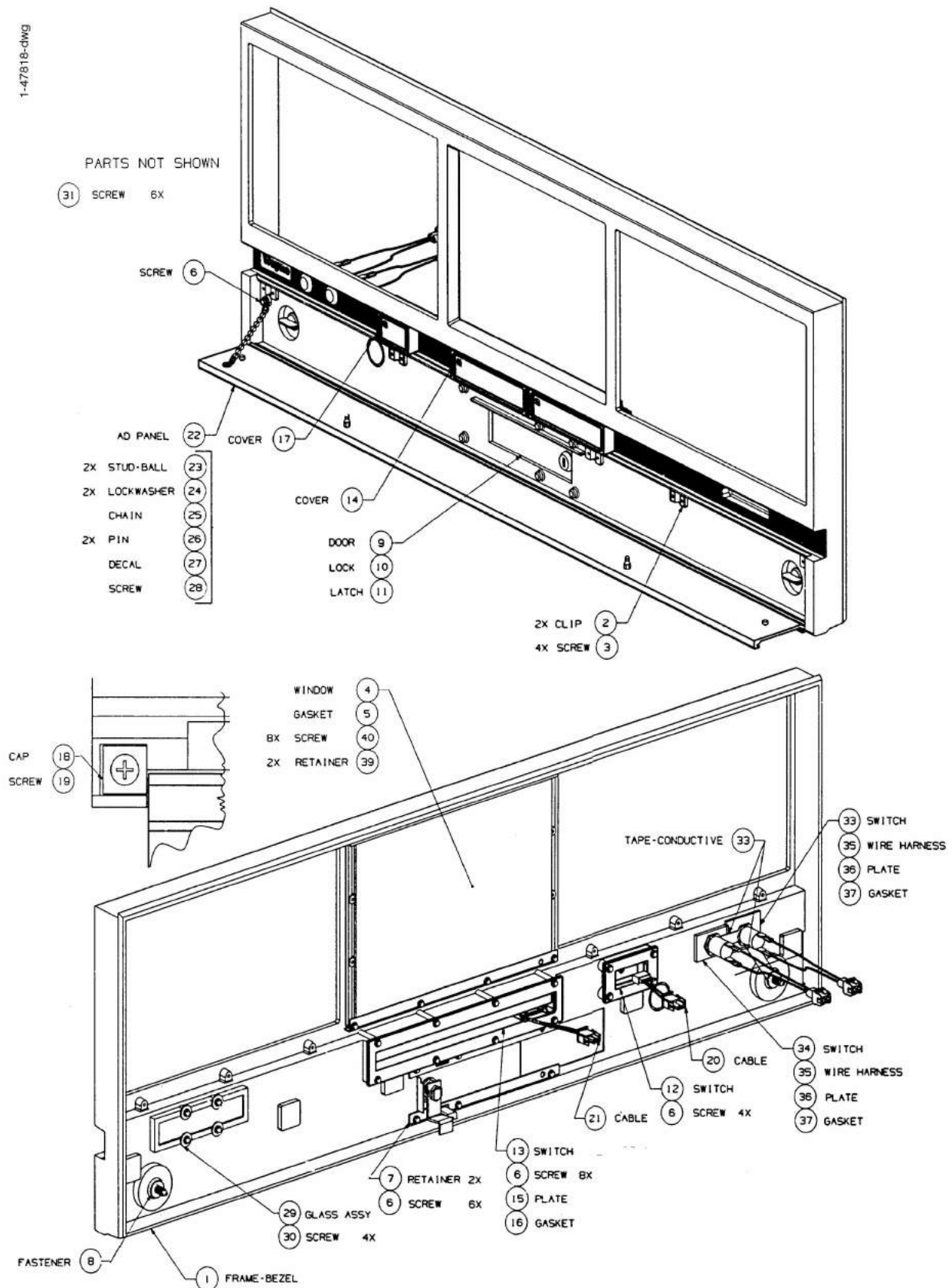
FIGURE 41. 1-47818-DWG - BEZEL MODULE
